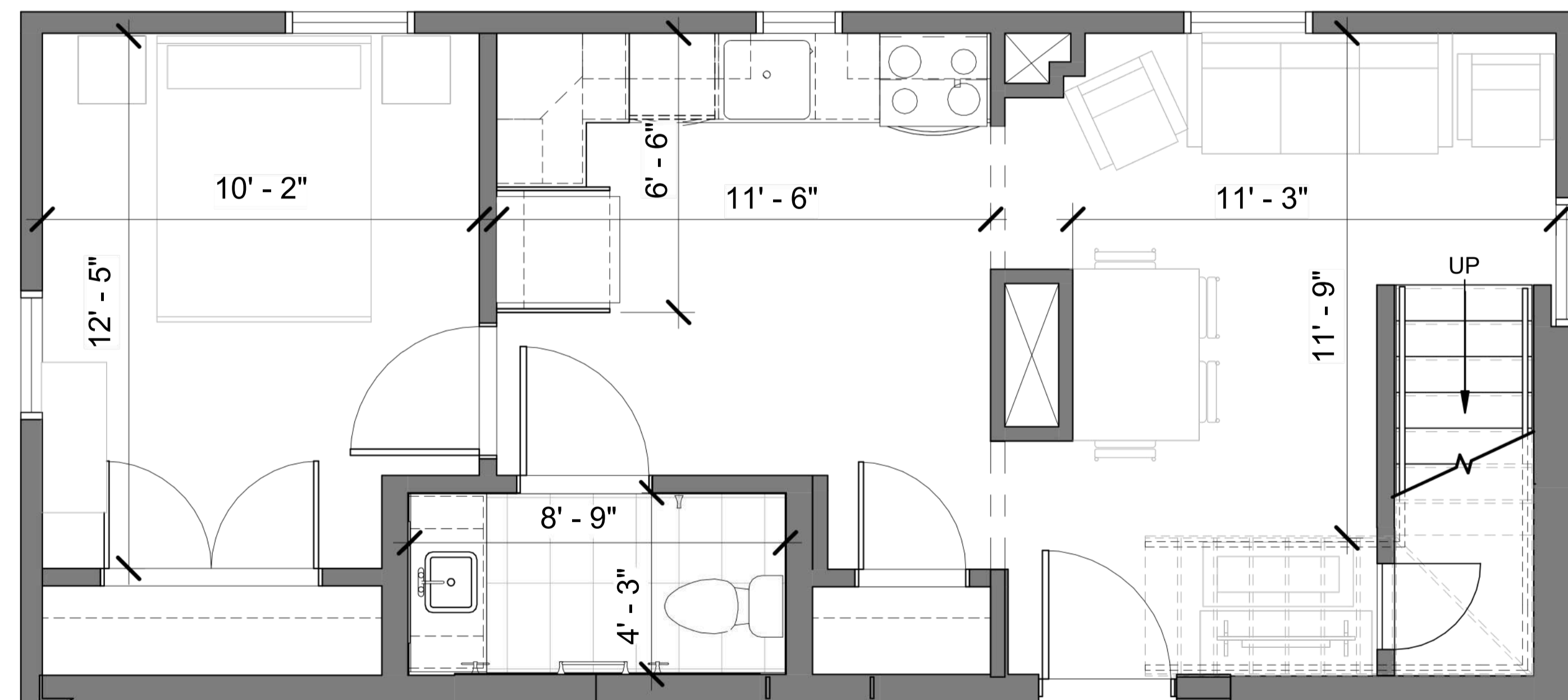
3BR TYPE E1 Level 1 Plan -1088 SF
