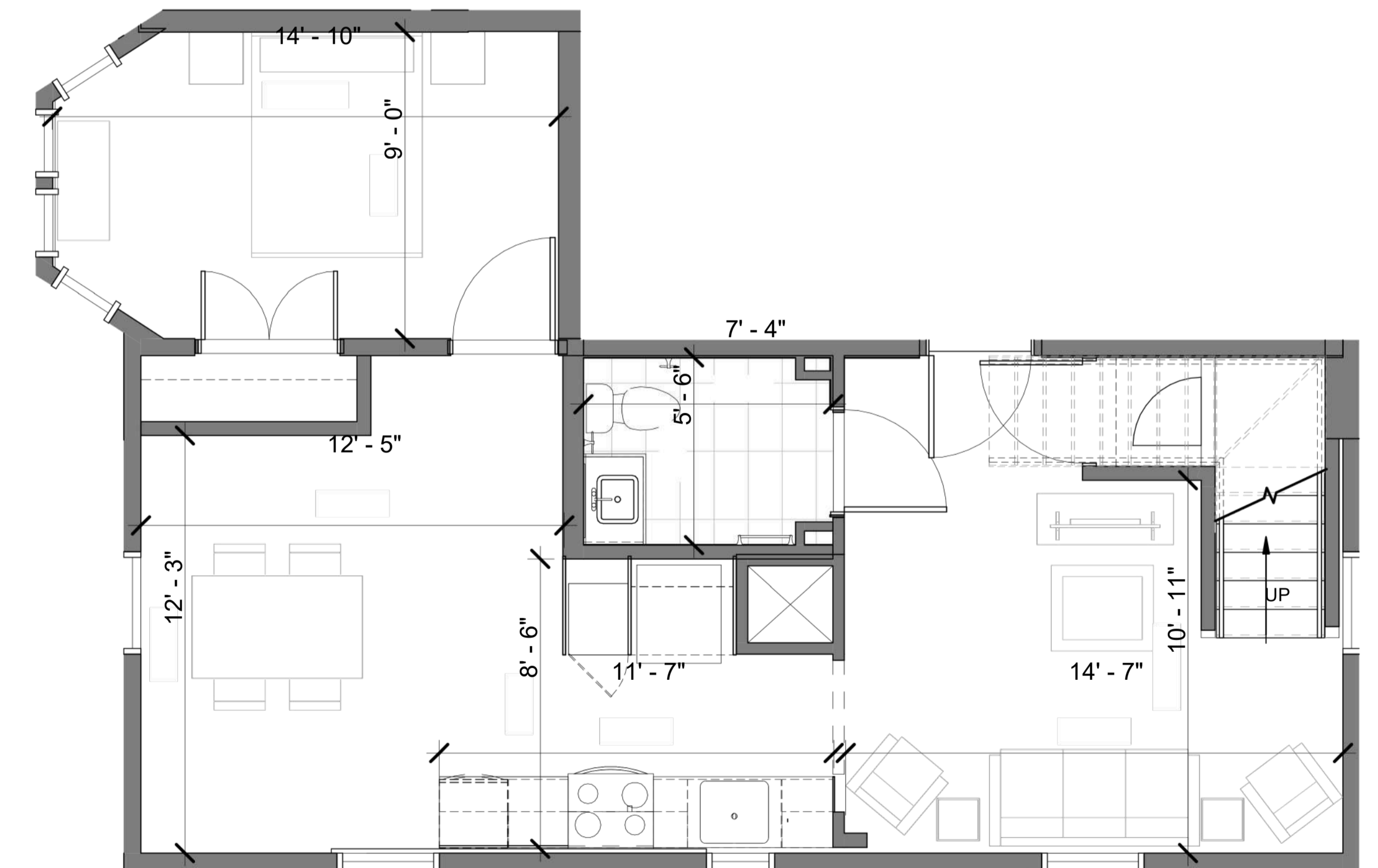
3BR TYPE E2 Level 1 Plan -957 SF
