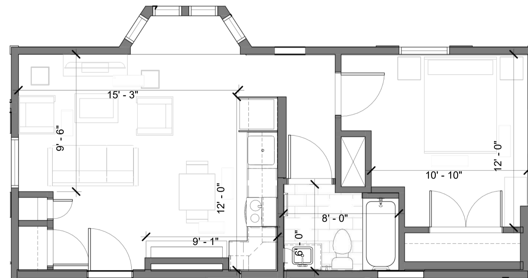
1BR TYPE E1 Plan -547 SF
