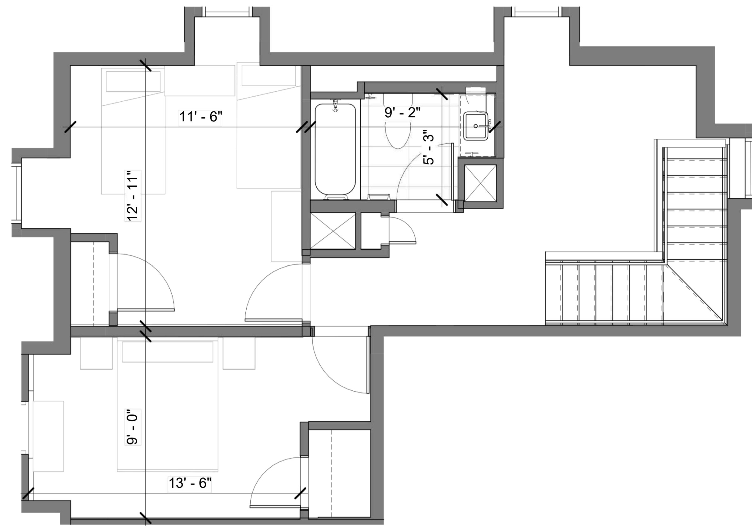
3BR TYPE E1 Level 2 Plan -1088 SF
