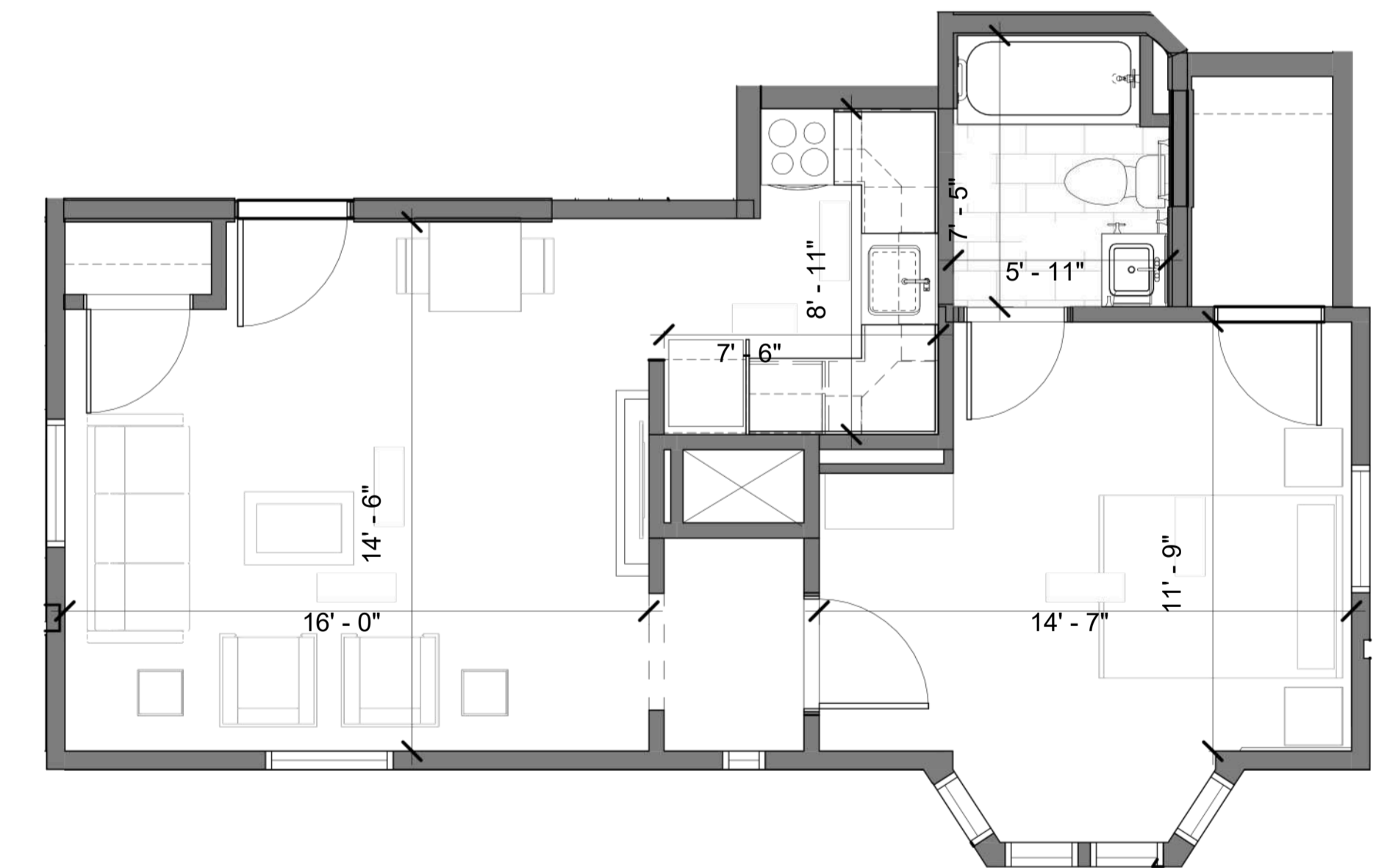
1BR TYPE E2 Plan -542 SF
